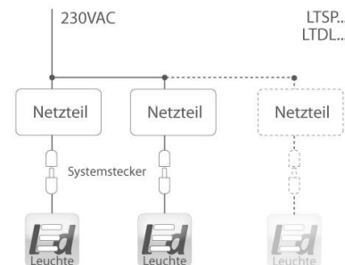
Schaltplan
