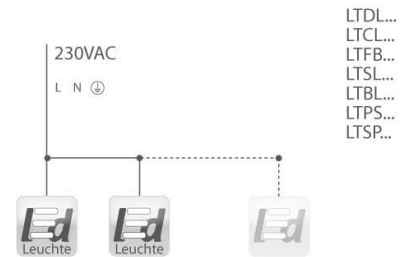
Schaltplan
